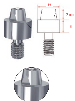
Caras planas que convierten el aditamento en no rotatorio
